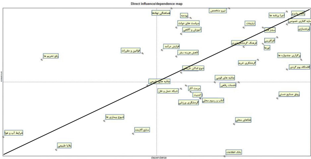
شکل ۵: پلان متغیرها
