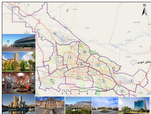
شکل ۱: نقشه محدوده مورد مطالعه
