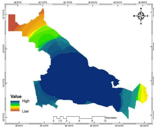
شکل ۶: نقشه همپوشانی بارش AHP
