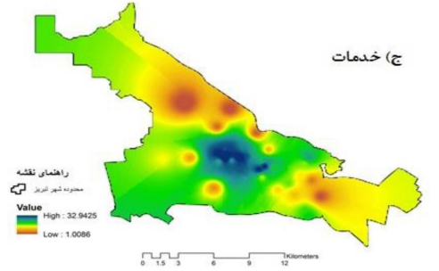
شکل ۵: نتایج مدل همپوشانی برای معیارهای اصلی
