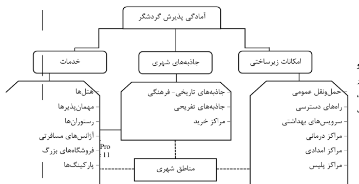
شکل ۳: طبقه‌بندی معیارهای پژوهش
